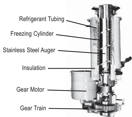
EVAPORATOR
